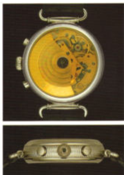
Die Rück- und Seitenansicht des Modells 6002 mit fein finisliertem Uhrwerk.
